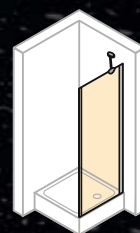
Bočná stena Šírka: 400–1000 mm Výška: 1600–2000 mm
