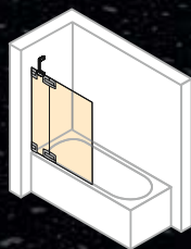
1-dielna s pevným segmentom
