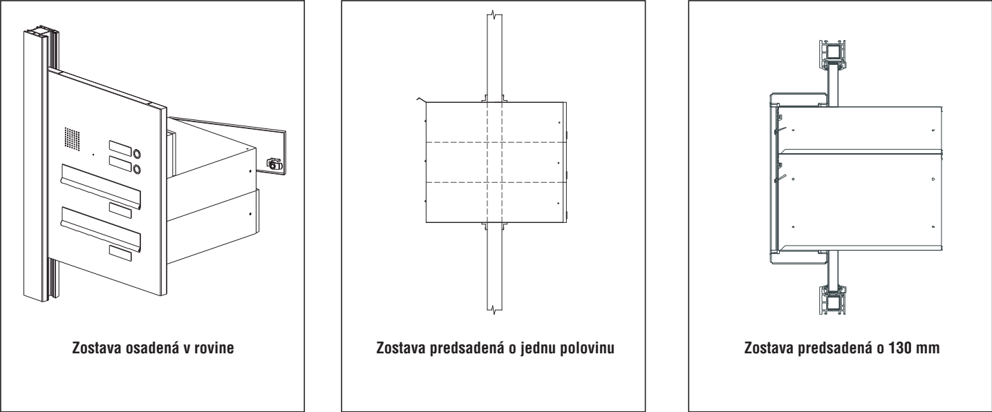
Čelná doska zateplená hr. 24 mm, umiestená v plastových profiloch. Doporučený presah čelnej dosky min. 30 mm
