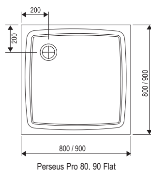
Perseus Pro 80, 90 Flat
