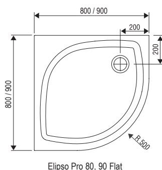
Elipso Pro 80, 90 Flat
