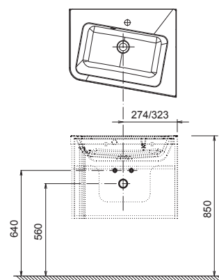
SD 10° rohová R
