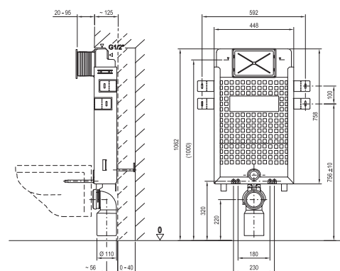
Predstavený inštalačný modul W
